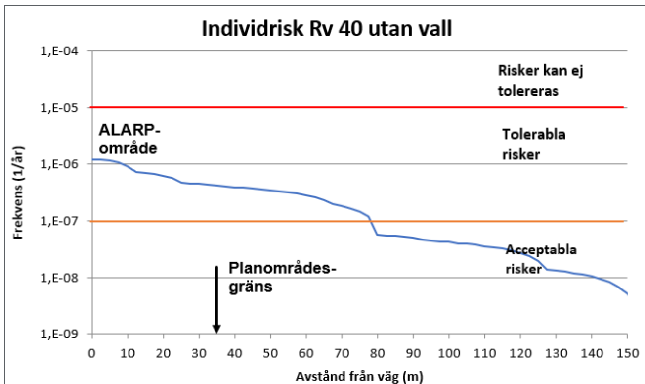
Figur 10 Individrisken längs riksväg 40 utan skyddsvall vid det studerade området.
