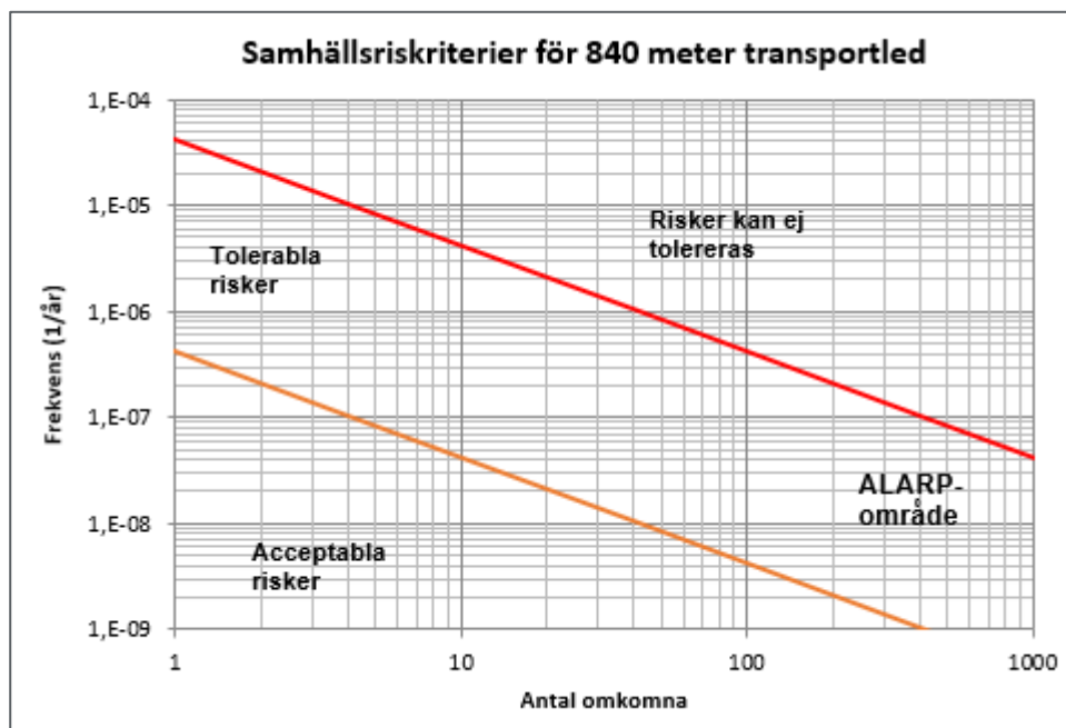
Figur 4. Riskkriterier omräknade till 840 meter enkelsidig bebyggelse.
