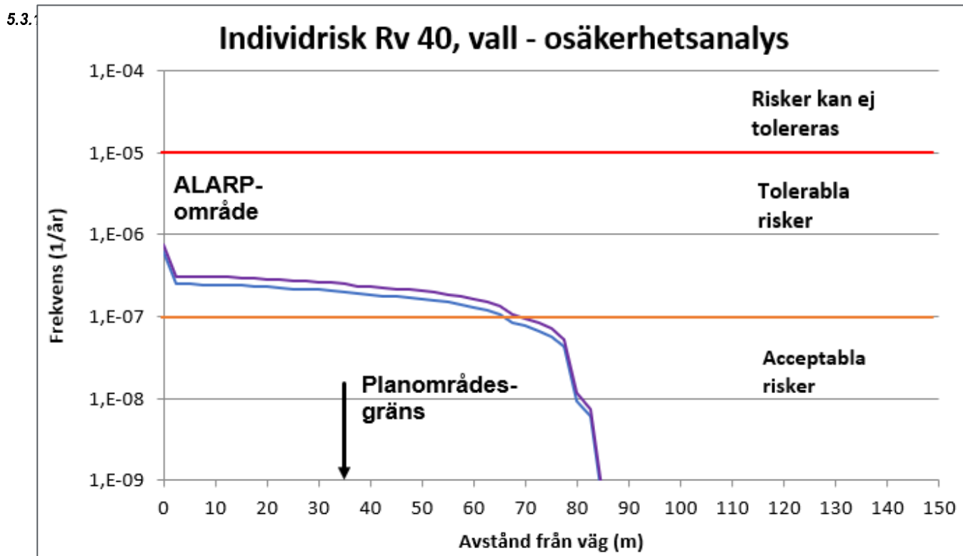
Figur 12. Osäkerhetsanalys för individrisken med skyddsvall, lila linje vid en ökning av antalet transporter av farligt gods med 25 %. Blå linje visar ursprungsberäkningen.
