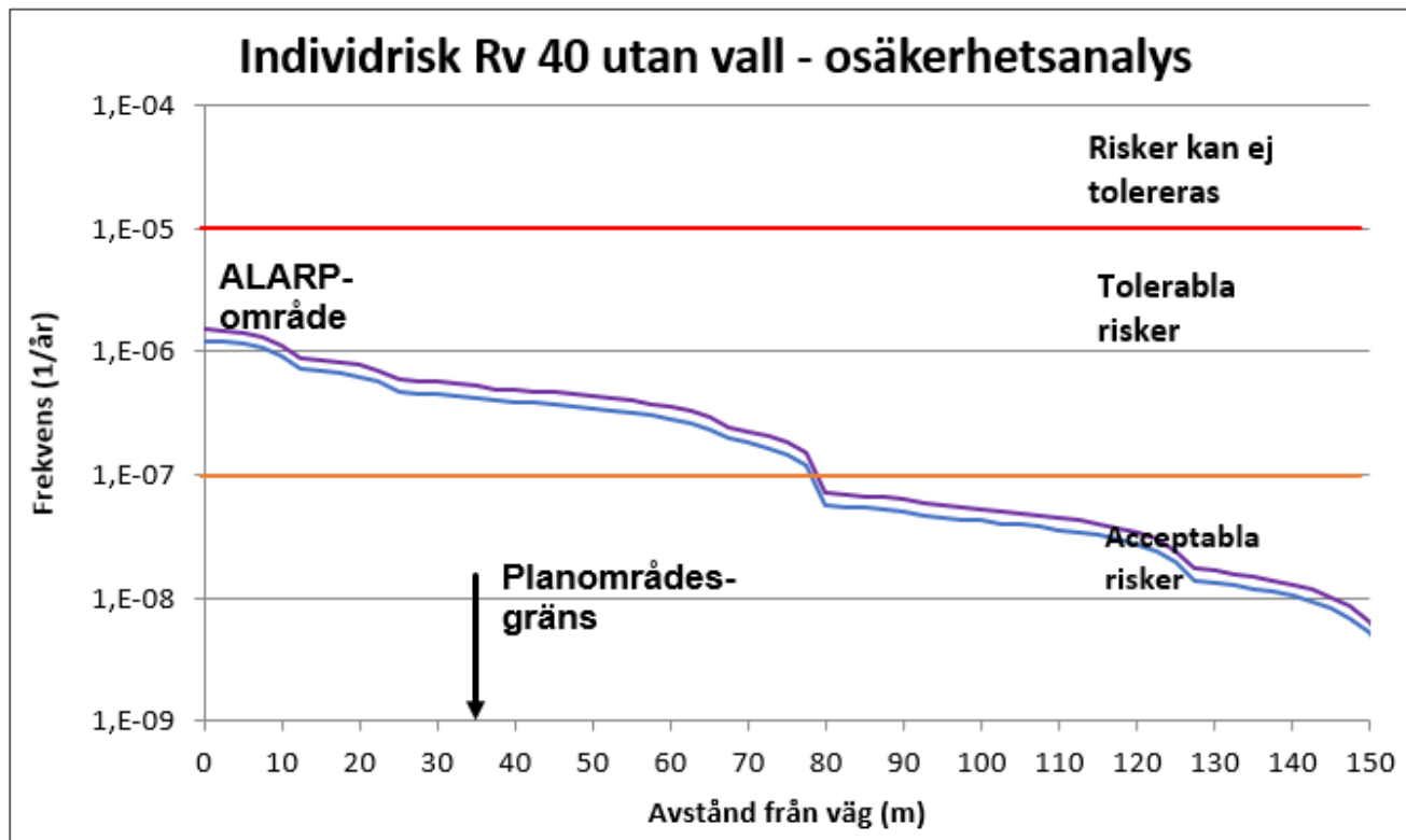
Figur 13 Osäkerhetsanalys för individrisken utan skyddsvall, lila linje vid en ökning av antalet transporter av farligt gods med 25 %. Blå linje visar ursprungsberäkningen.
