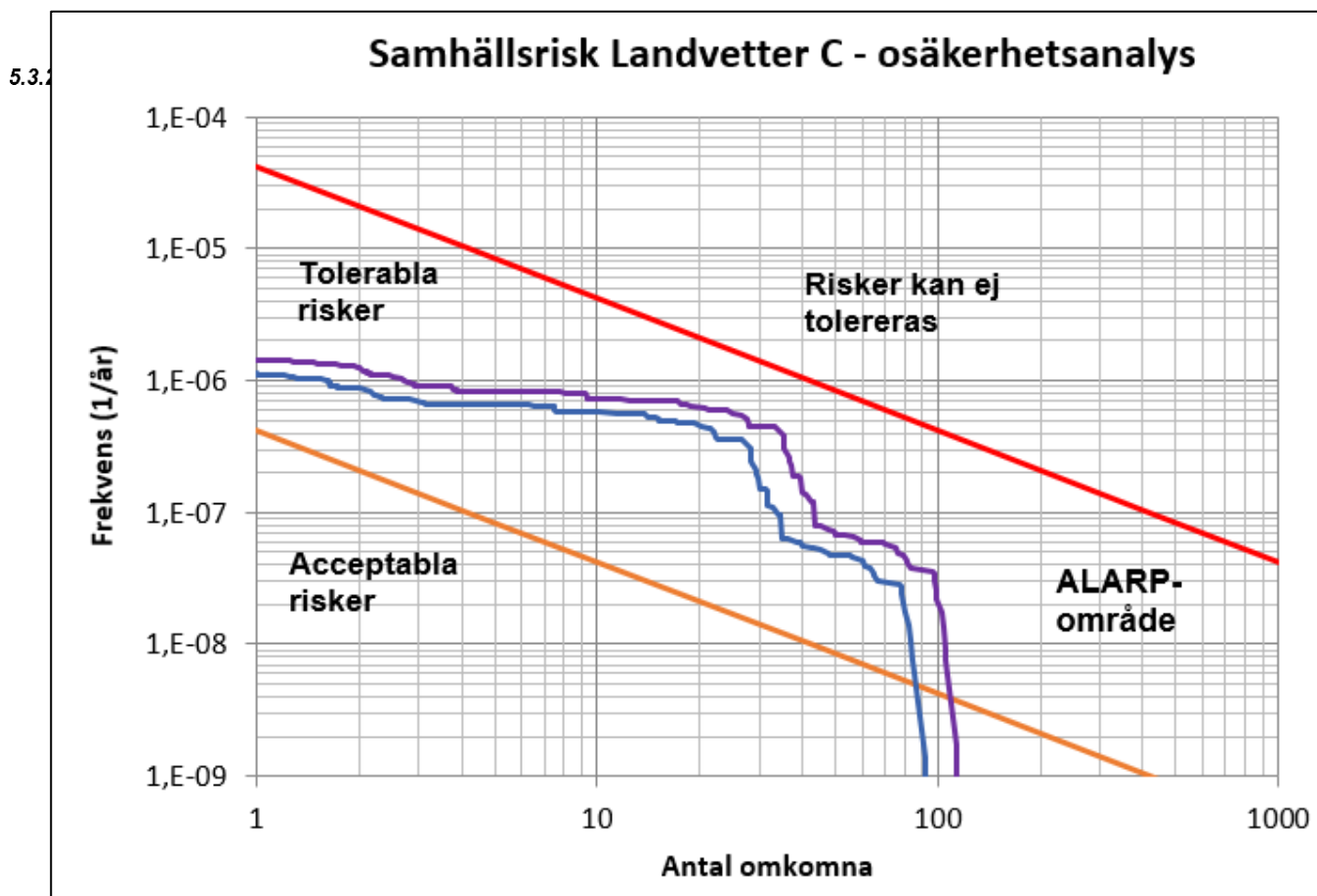
Figur 14. Osäkerhetsanalys för samhällsrisken för en ökning av antalet transporter med farligt gods samt ökning av antalet personer med 25 % (lila linje). Blå linje visar ursprungsberäkningen.
