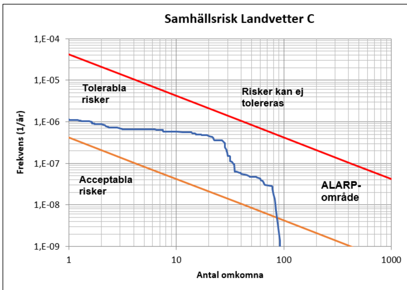
Figur 11. Samhällsrisken för etablering i Landvetter centrum.
